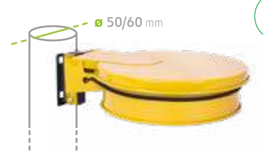
Adattatore per palo rotondo Ø 50/60 mm Adapter for Ø 50/60 mm post
